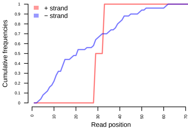
C>T
