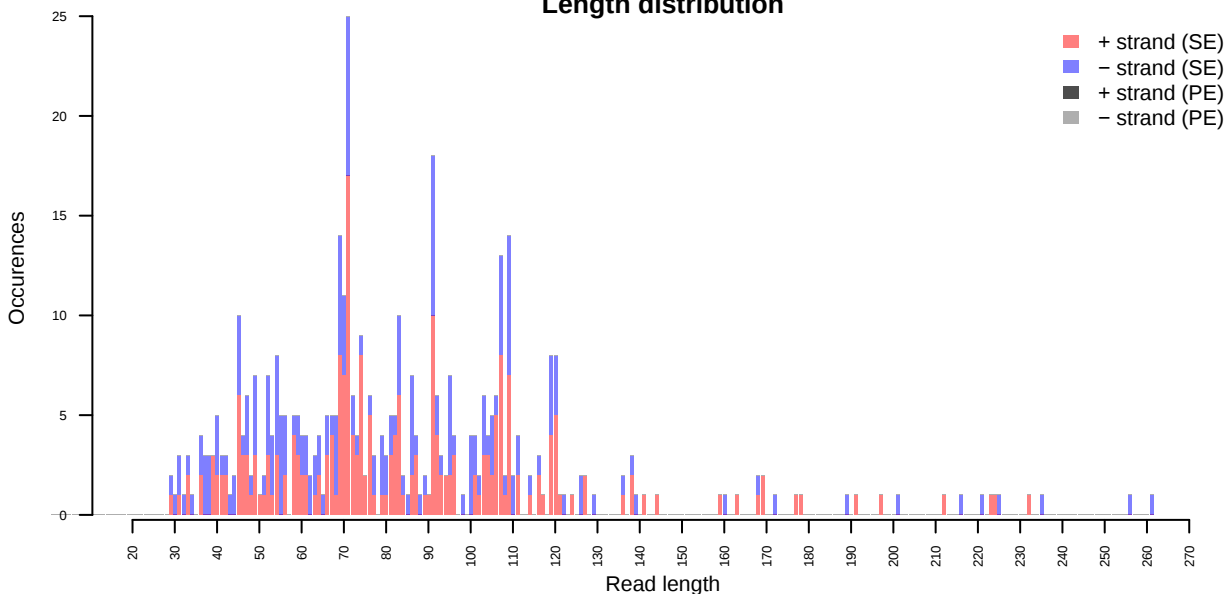
C>T
