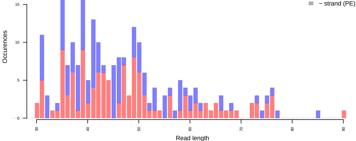
C>T
