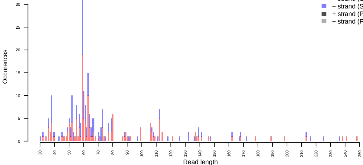
C>T
