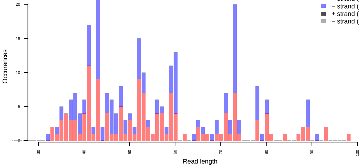
C>T
