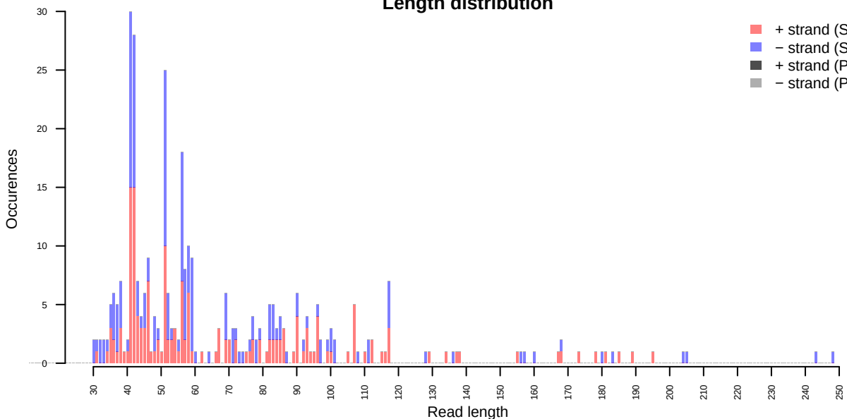
C>T
