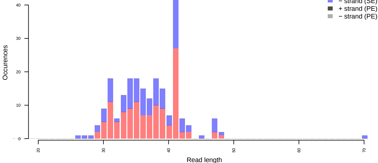
C>T
