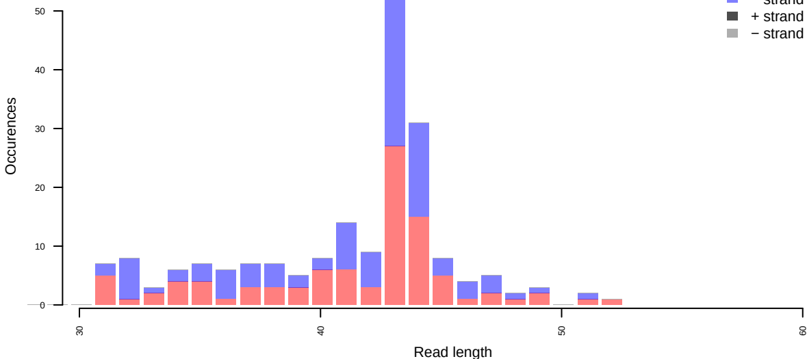
C>T
